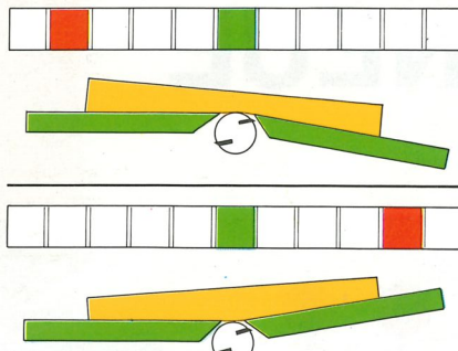
Hohl-Spitzfugen-Anzeige 2
