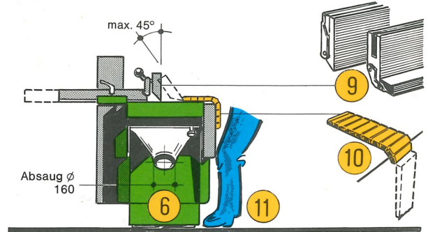
Autom. Messerwellen-Bremse 4
