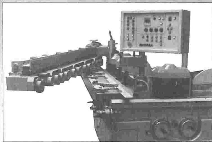
Frasenheiten UF, Gegenanschlag, weggeschwenkter Vorschub (Hier Modell UF-S)
